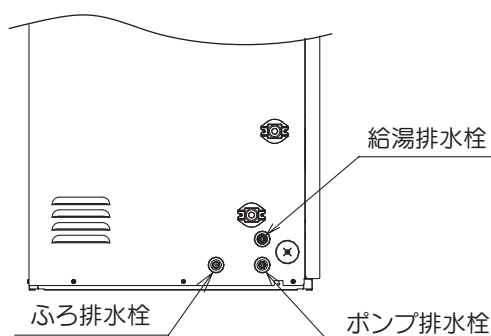
排水栓位置図
