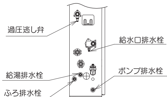
排水栓位置図
